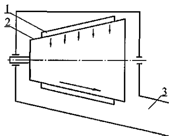
Рис. 5. Схема барабанно-конусного робочого органу:
