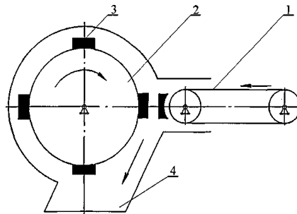
Рис. 4. Схема барабанного подрібнювального апарата:
