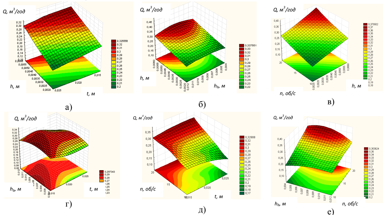
Рис. 2. Поверхні відгуку залежностей: а – Q = f(h, t) ; б) – Q = f(h, h_b) ; в) – Q = f(n, h) ; г) – Q = f(h_b, t) ; д) – Q = f(n, t) ; е) – Q = f(h_b, n)
