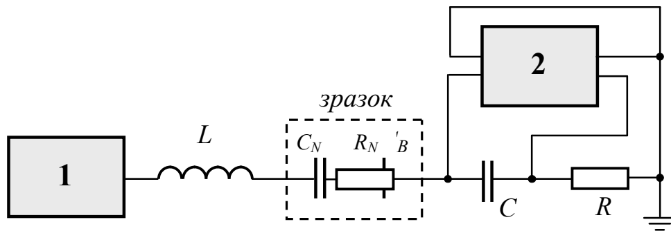
Рис. 4. Блок-схема методу нелінійного діелектричного резонансу [12], 1 – генератор; 2 – осцилоскоп
