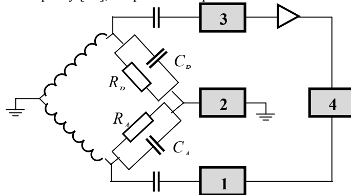
Рис. 3. Блок-схема пристрою для вимірювання нелінійної діелектричної константи \Delta\varepsilon(\omega) , 1 – низьковольтний і високочастотний генератор; 2 – високовольтний низькочастотний генератор; 3 – демодулятор; 4 – осцилоскоп
