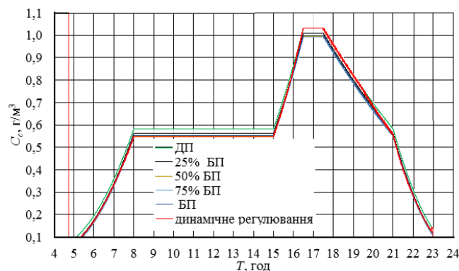
Рис. 7. Залежність концентрації сажі C_s від години доби T при роботі дизельного генератора
