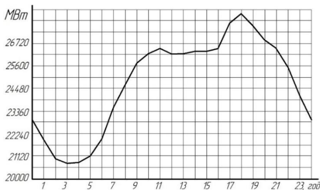
Рис. 1. Графік середнього споживання електроенергії в Україні в робочі дні за листопад
