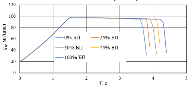
Рис. 8. Залежність циклової подачі суміші палив q_{ц} з різним відсотковим складом від часу T при розгоні колінчастого валу дизеля
