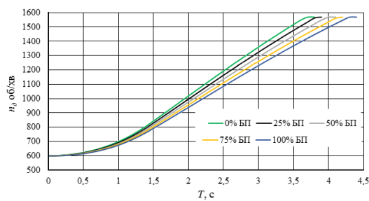
Рис. 9. Залежність частоти обертання колінчастого валу n_d від часу T при розгоні його на суміші палив різного відсоткового складу
