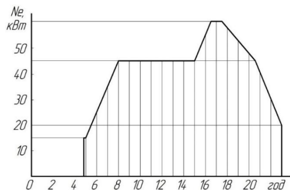
Рис. 2. Зміна навантаження на дизельний генератор
