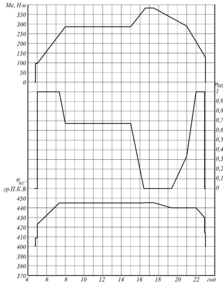
Рис. 6. Графік залежності ефективного крутного моменту M_e , відсоткового складу суміші палив n_{БП} та значення кута повороту колінчастого валу при закінченні горіння суміші палив \varphi_{32} в циліндрі дизеля від години доби
