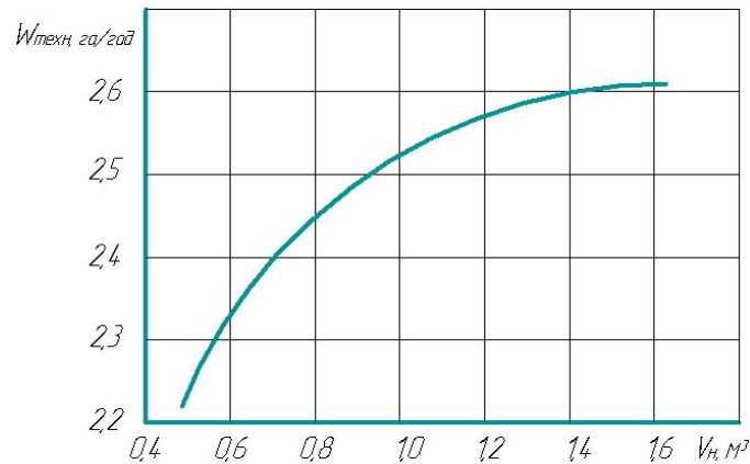
Рис. 1. Залежність технічної продуктивності посівного агрегату W_{\text{техн}} , скомплектованого на базі сівалки АСТРА СЗ-3,6А в залежності від можливої зміни об'єму насінневого ящика V_n
