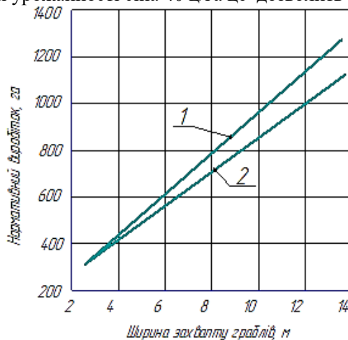
Рис.3. Залежності впливу ширини захвату граблів на їх нормативний річний виробіток при довжині гонів: 1- 1000, 2-400 м
