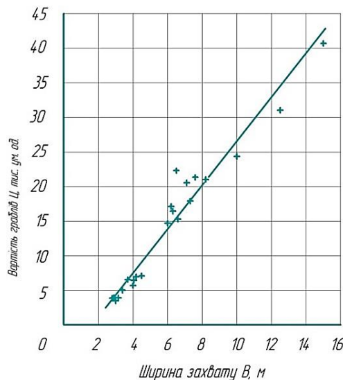
Рис. 1. Залежність зміни вартості граблів з керованими граблями Ц від ширини захвату В
